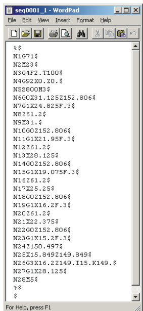
Slika 8. Postupak automatizovanog generisanja putanje alata za zahvat grubog struganja podoperacije 30/1
